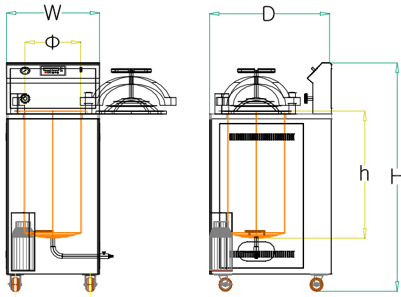
*Auto Clave, Dimensions DK-AC60
